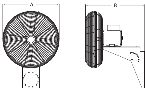
Figura 2 — Dimensiones del Modelo para Lugares Peligrosos
