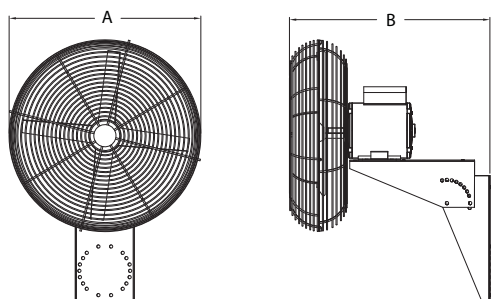
Figure 2 — Dimensions Zone dangereuse
